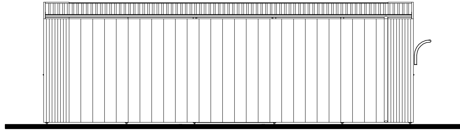
elewacja południowa
