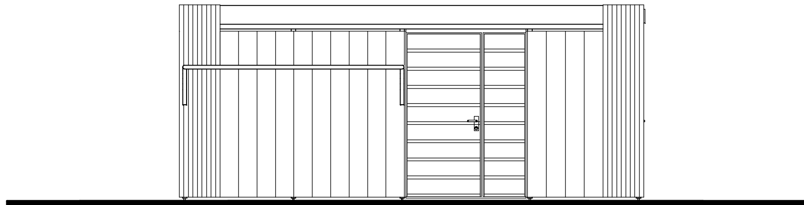
elewacja wschodnia
